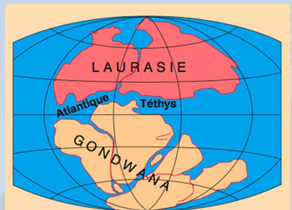
Disposition des continents et des océans vers le milieu du Jurassique, il y a 160 millions d'années (ou 160 mille millénaires)
